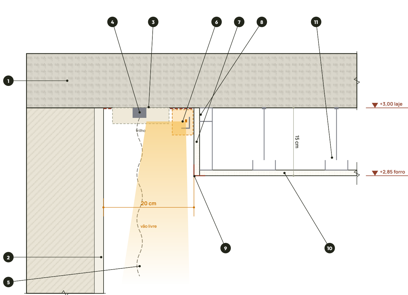
C1 Corte do cortineiro • suite master escala 1:5 · entreforro 15 cm
