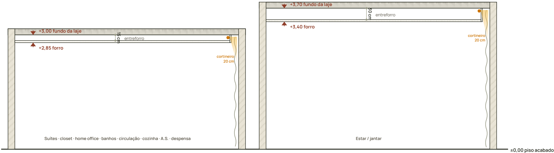
ESQUEMA DE NÍVEIS corte esquemático - alturas do piso acabado ao forro e ao fundo da laje (DWG) - vertical 1:60, horizontal sem escala
