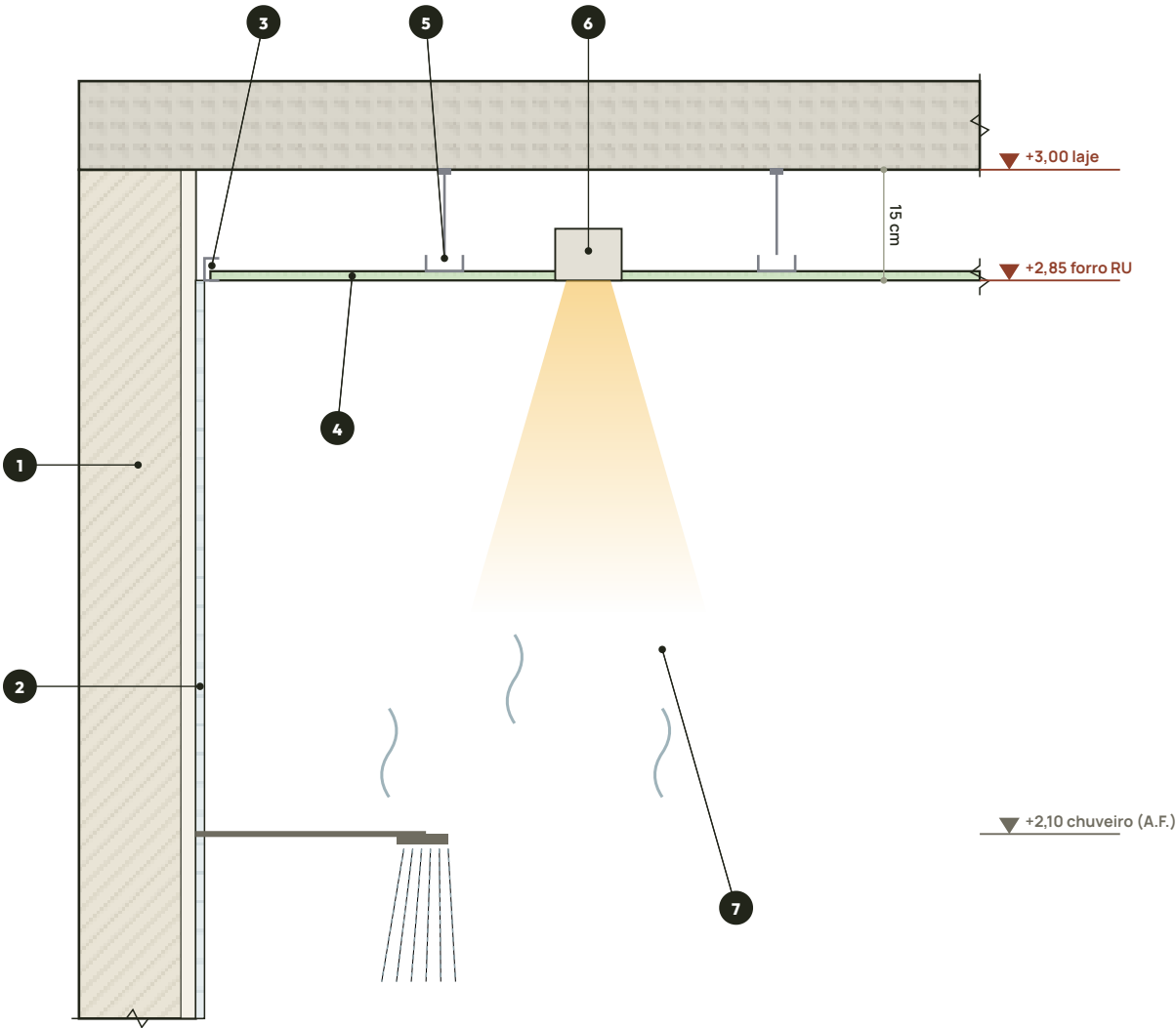
B1 Corte típico · forro RU no banho escala 1:10 · vale para os 4 banhos
