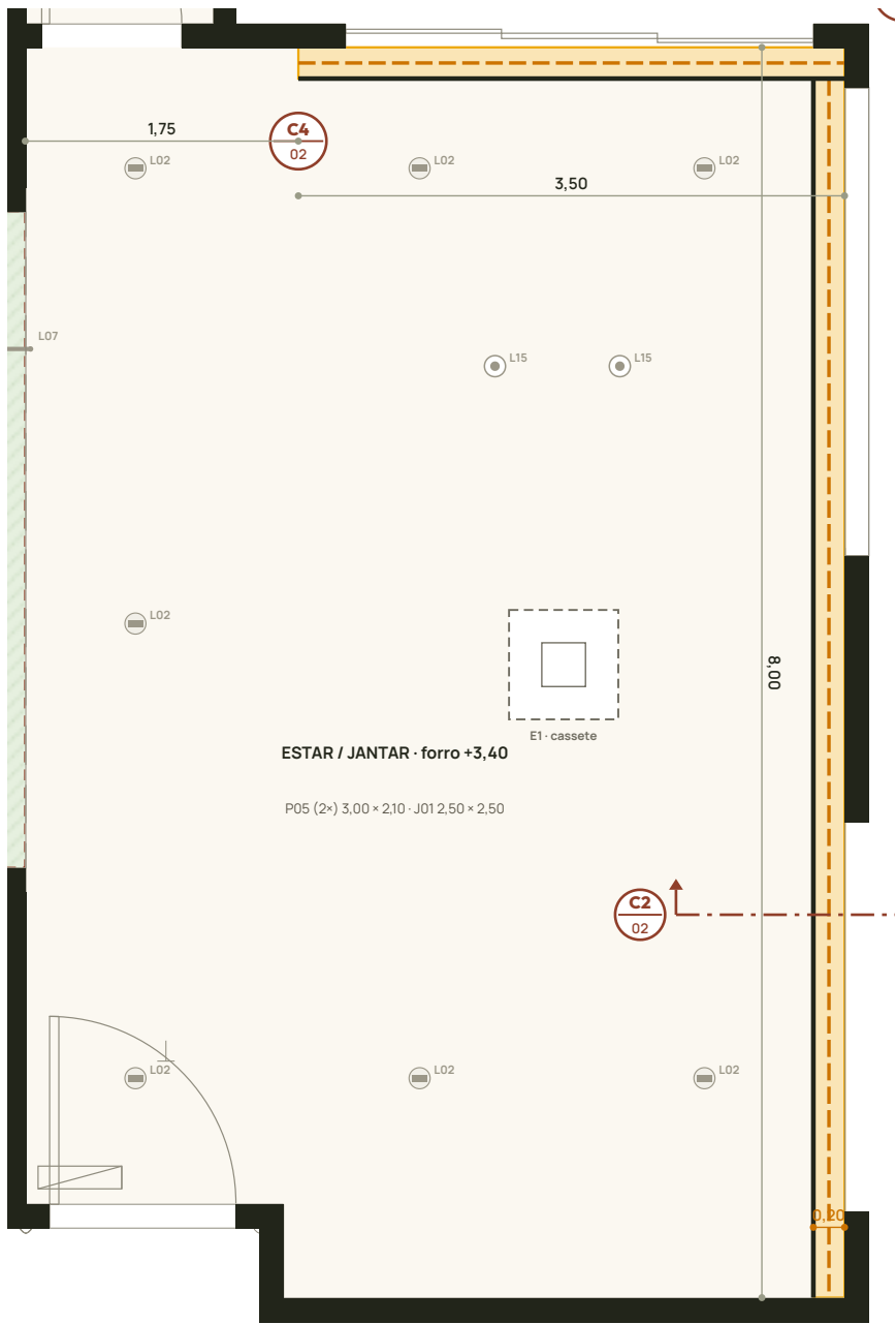
CT2 Cortineiro • estar / jantar planta 1:50 · L09 TuboLED
