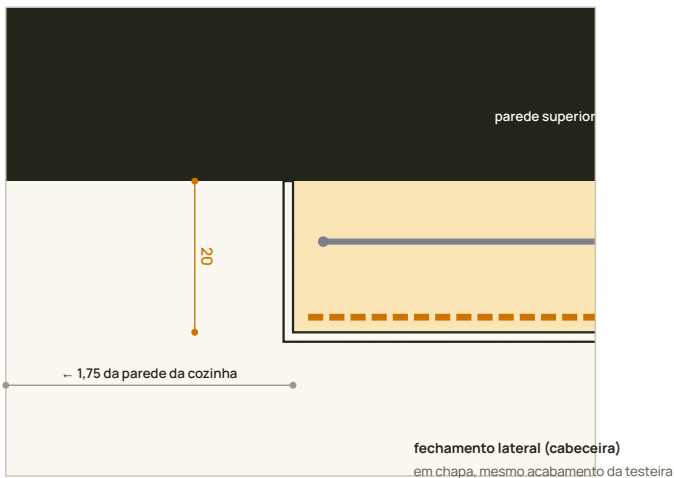
C4 Cabeceira • CT2 planta 1:10
