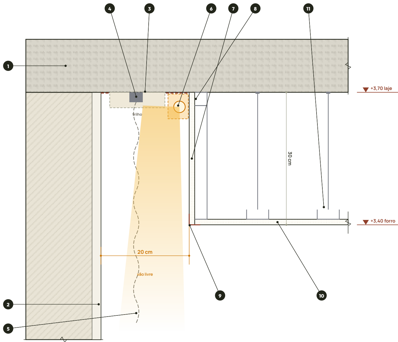
C2 Corte do cortineiro • estar / jantar escala 1:5 · entreforro 30 cm
