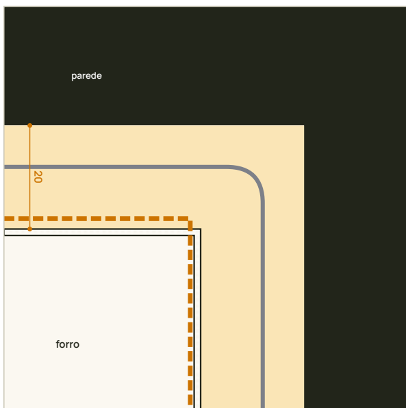
C3 Canto em L • CT2 planta 1:10
