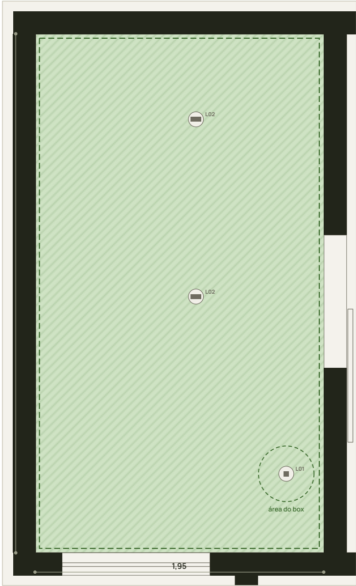
B Banho Suíte Master planta 1:25 · 6,83 m² · forro +2,85 · placa RU
