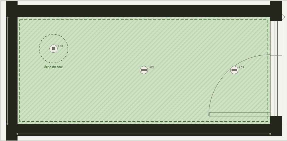
B Banho 4 planta 1:25 · 4,62 m² · forro +2,85 · placa RU
